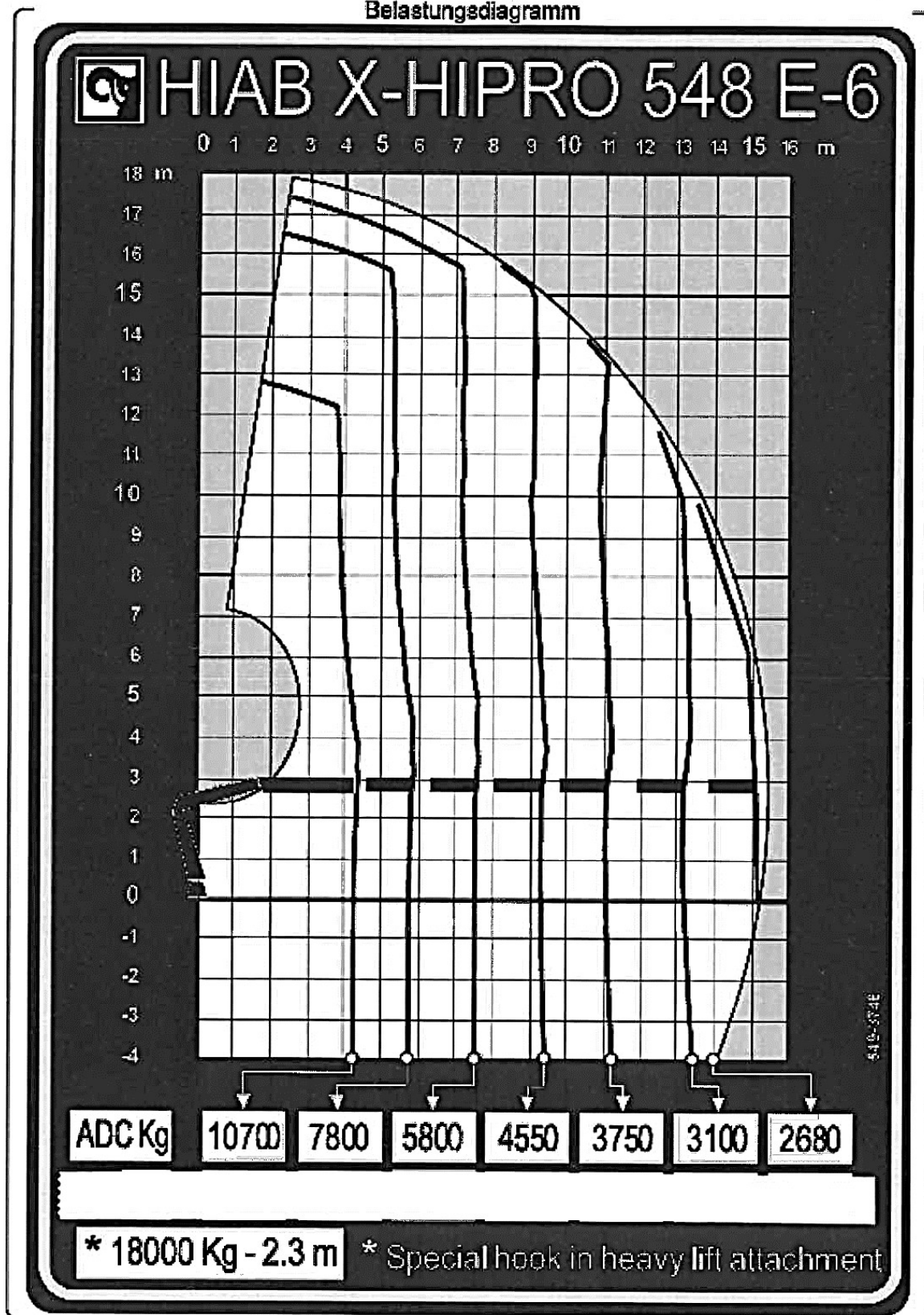
Belastungsdiagramm
